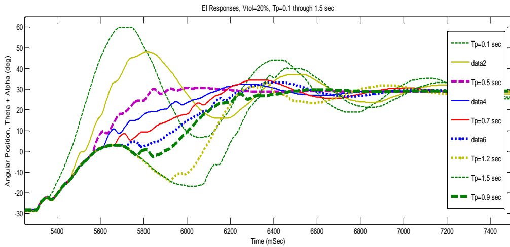
Figure 6: Actual Res. to 20% EI – Experimental
