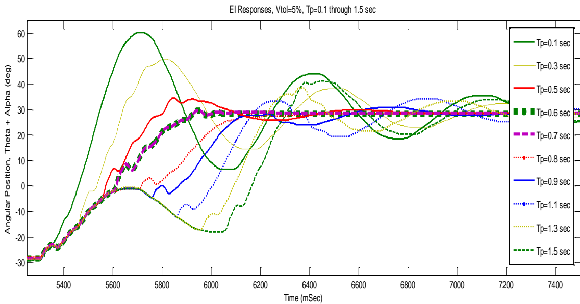
Figure 5: Actual Res. to 5% EI – Experimental
