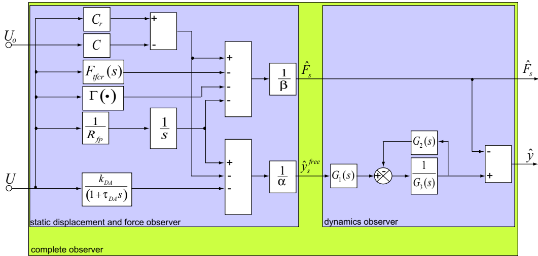
Fig. 3. Block diagram of the actual observer.
